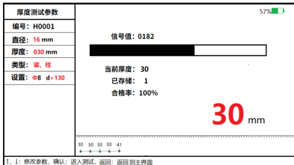
图 3-2 厚度测试界面
