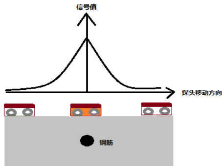
图 2-1 测试原理图
