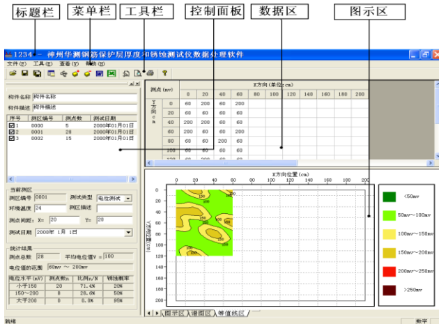
图 6-15 软件总体界面
