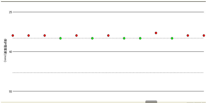
图 6-12 钢筋保护层厚度测试、JGJ 测试的图示
