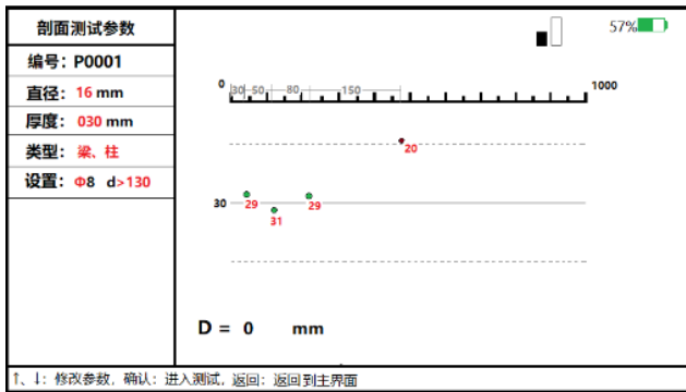
图 3-3 剖面测试界面
