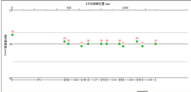
图 6-13 剖面测试图示
