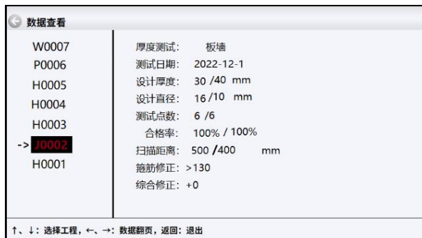
图 3-12 JGJ 扫描数据
