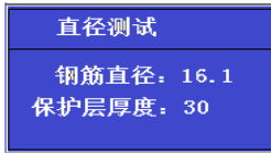
图 3-7 直径测试结果
